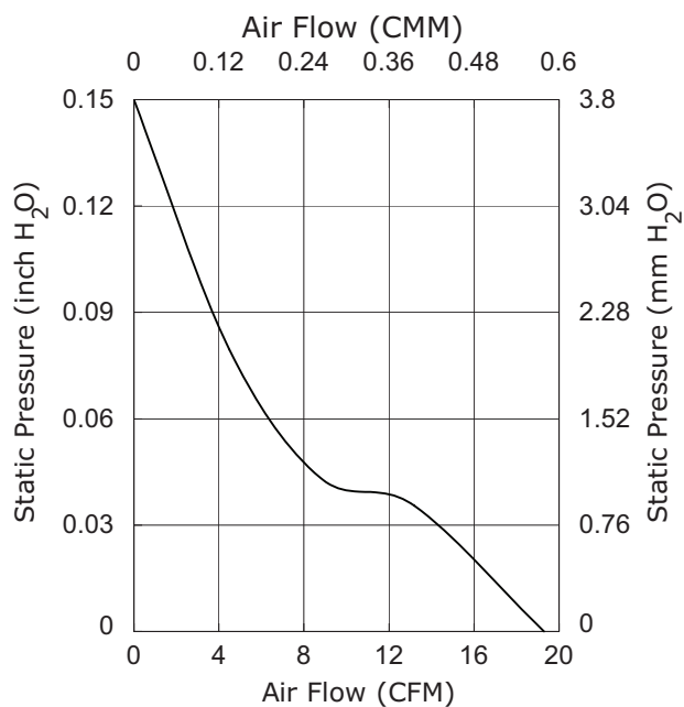
CFM-6025V-138-220
