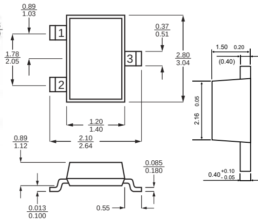
SOT-23
